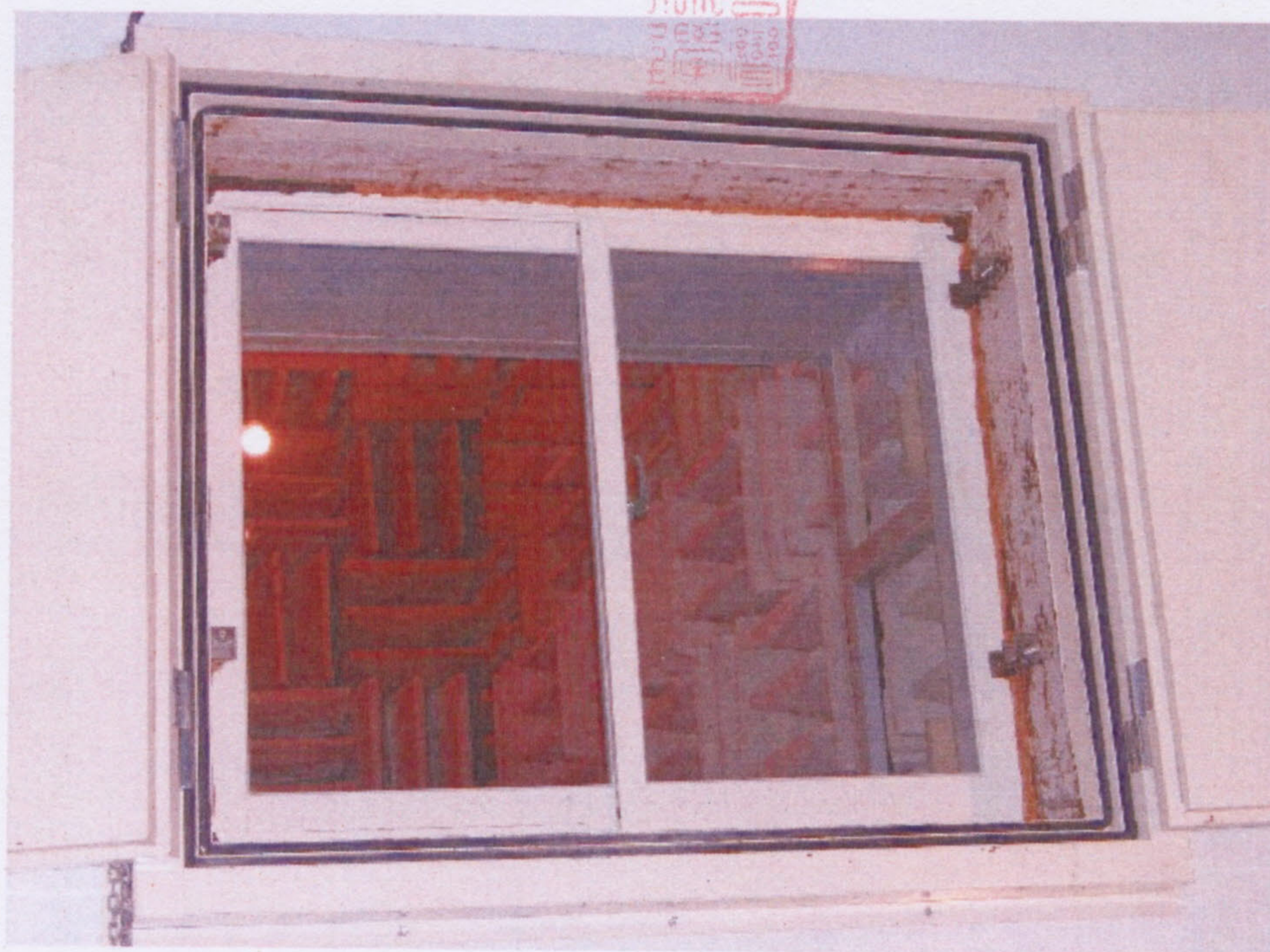
圖 2 試樣佈置圖 (迴響室)
