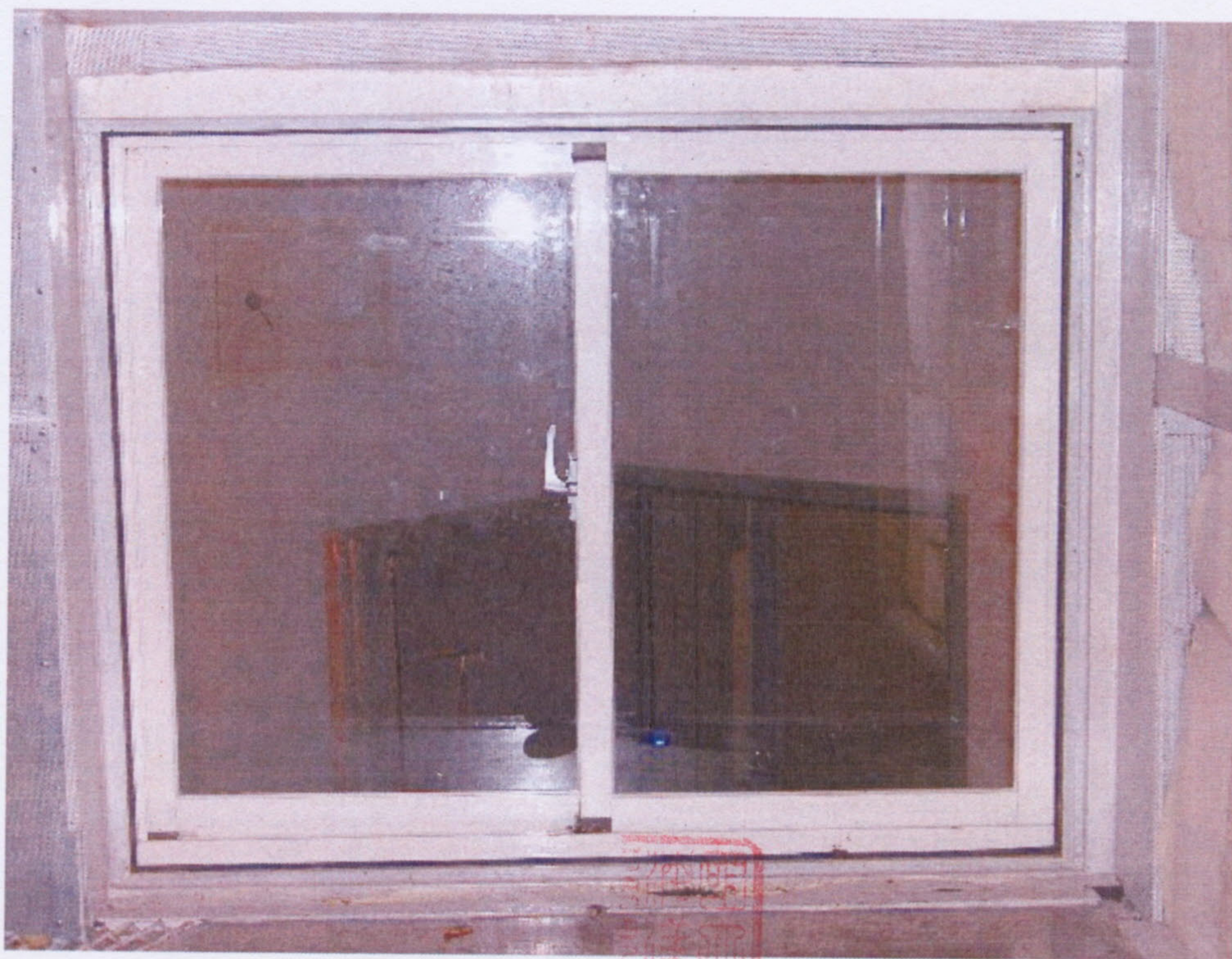
圖 1 試樣佈置圖 (無響室)
